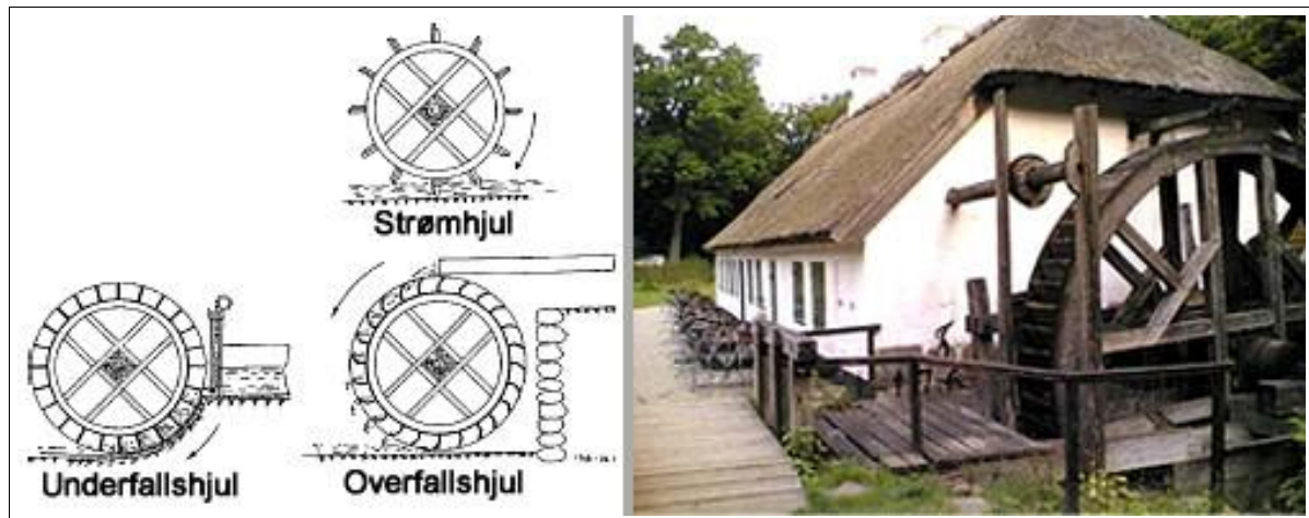
Til høyre Hammermøllen i Hellebæk med sine vannhjul. Hjulene er en variant av underfallshjulet.
