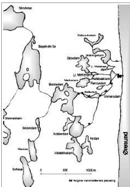
Geværfabrikkens vannkraftsystem. Hellebækken renner fra Bondedammen til Øresund. Den er ca. 1 kilometer lang og har en fallhøyde på ca. 20 meter. Derfor kunne den nokså begrenset vannmengde drive en rekke møller på denne korte strekningen. De mange sjøer som heter noe med "dam" er alle kunstig anlagt.
