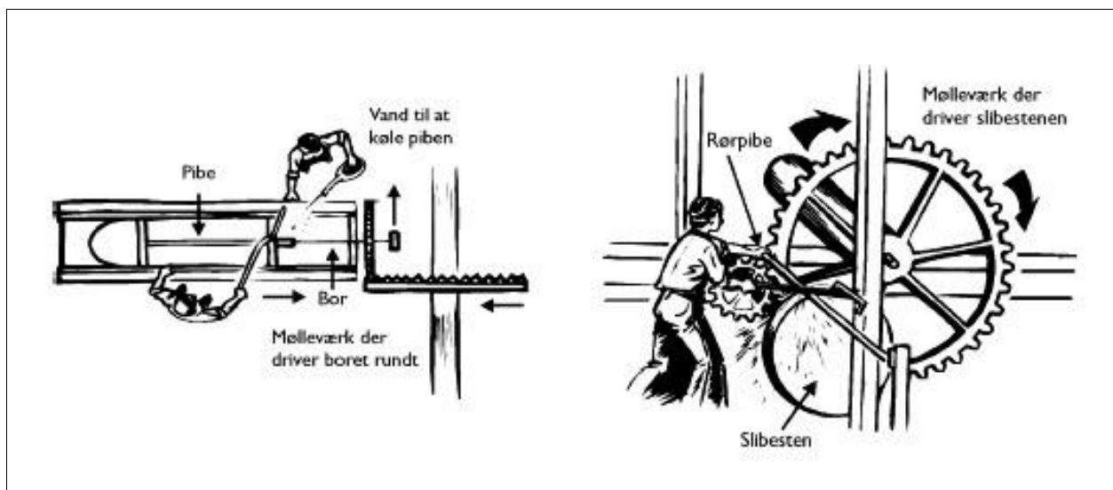
T. v. Boremøllen. - T. h. Slipemøllen.
