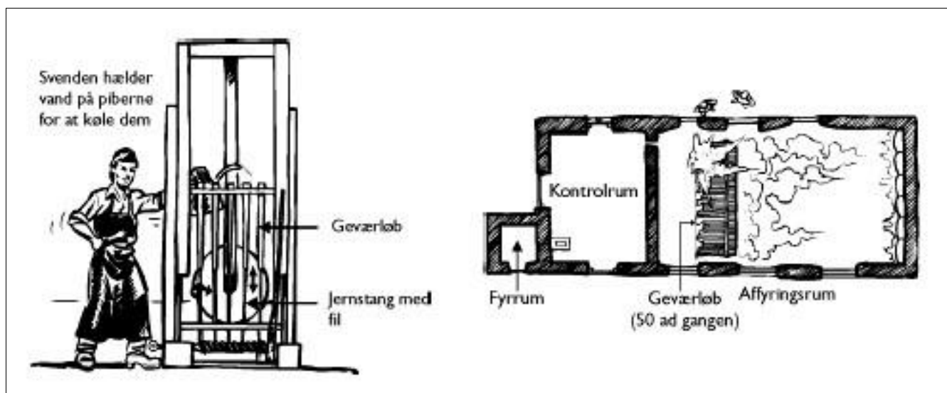
T. v. Trekning av geværløpene. - T. h. Styrkeprøven.
