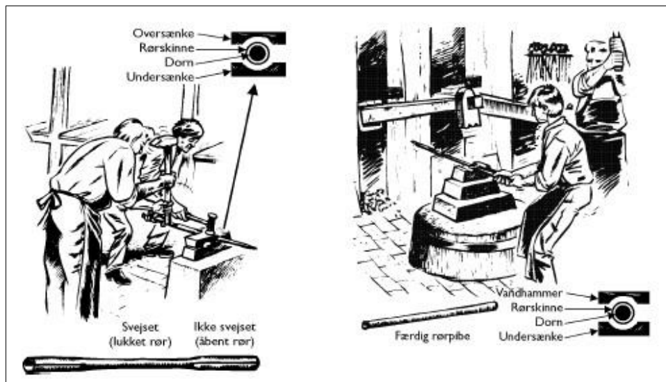
T. v. Rørskinnen sveises til et rør. - T. h. Sveising under vannhammeren.
