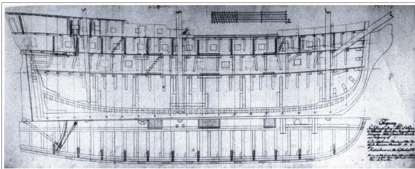
Gennemsnitstegning til DEN GODE HENSIGT efter de reviderede tegninger, som var en følge af statens overtagelse af byggesagen.
